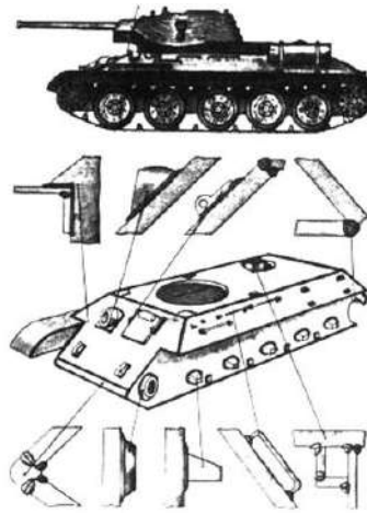
Рис. 1.44. Основные сварные узлы танка Т-34
